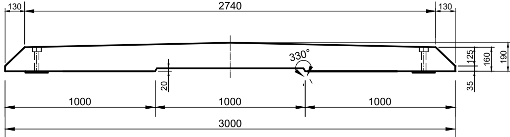
VORDERANSICHT
