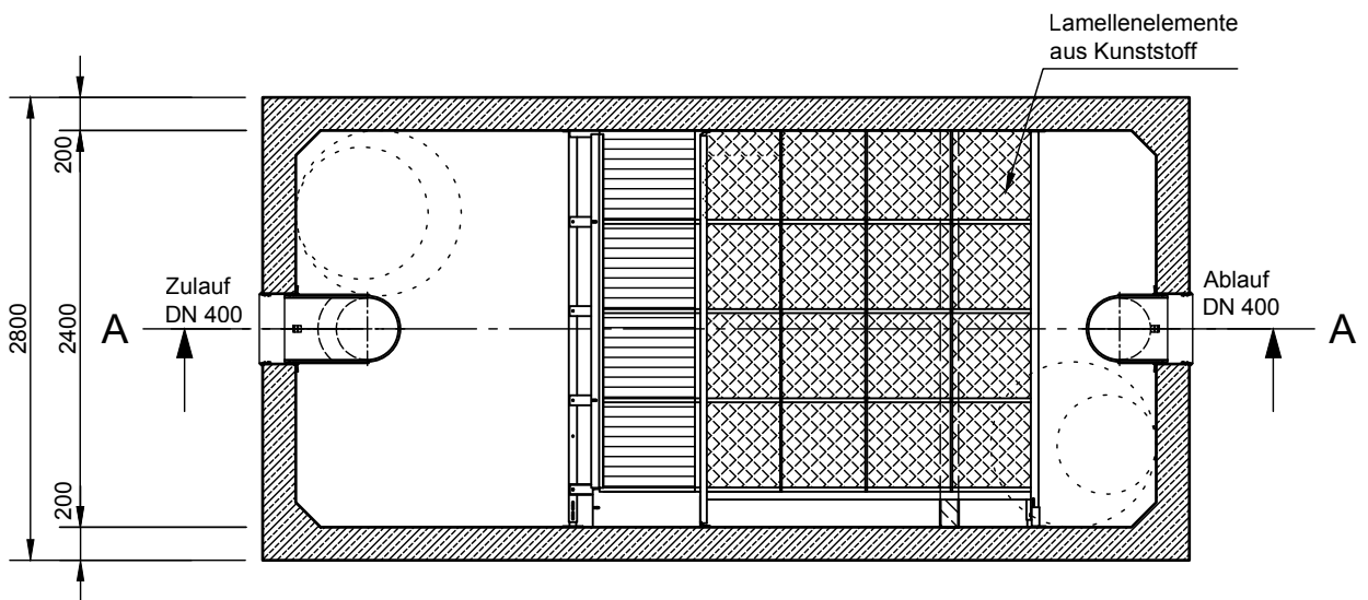
Grundriss
