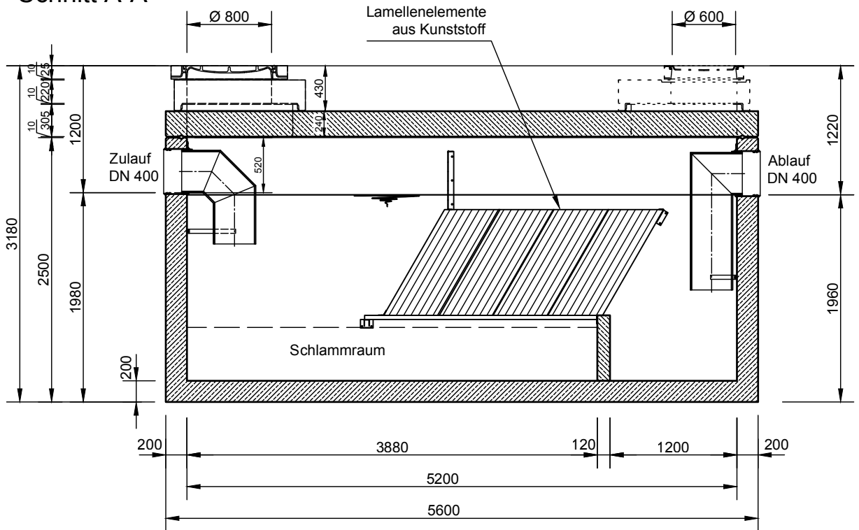
Schnitt A-A
