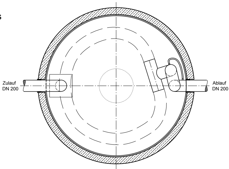
Grundriss
