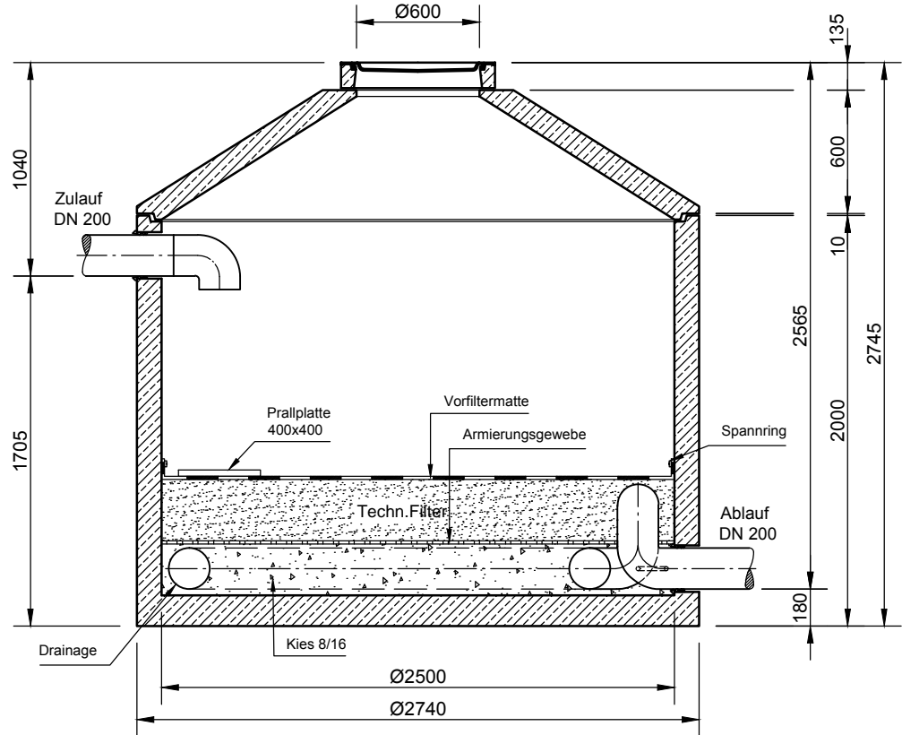
Schnitt
