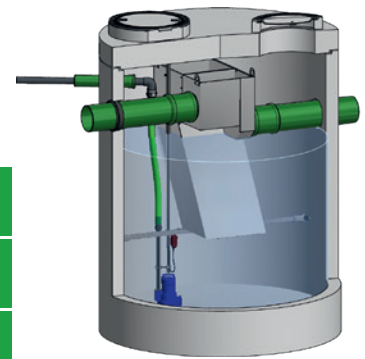
Mall-Lamellenklärer ViaKan ohne Dauerstau
