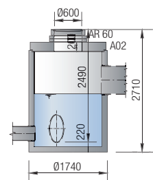
Vereinigungsbauwerk ViaPool
