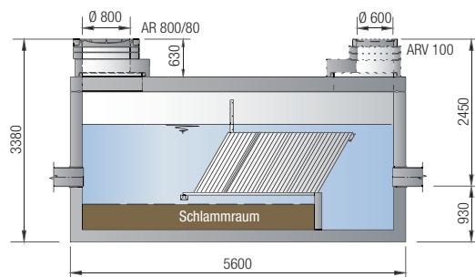
Lamellenklärer ViaTub II / III
