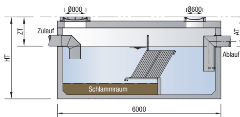
Lamellenklärer ViaTub
