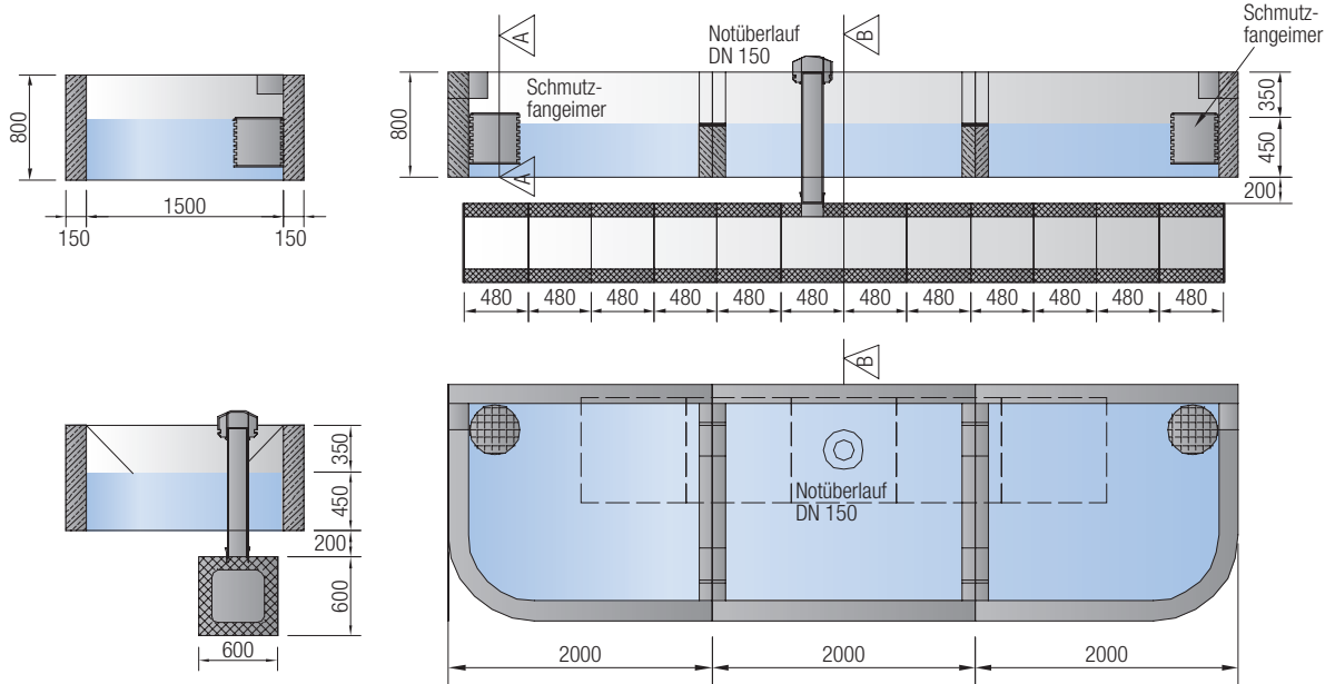
Tiefbeet-Bodenfilter Innodrain
