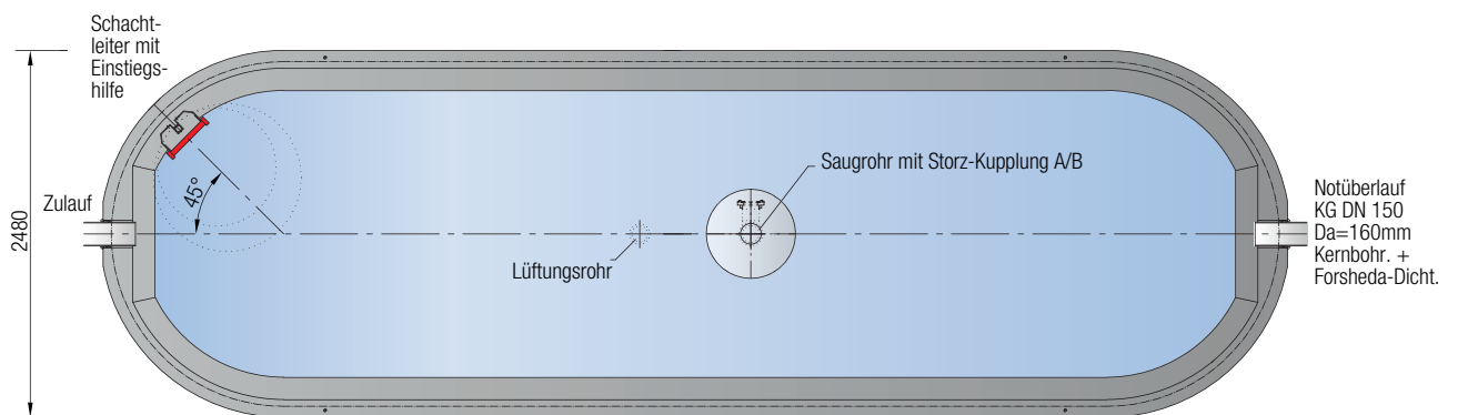
Löschwasserbehälter
