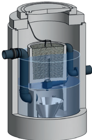
ViaPlus 500
