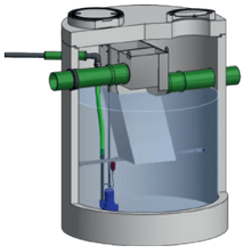
Mall-Lamellenklärer ViaKan ohne Dauerstau
