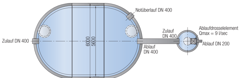
Regenrückhaltebecken
