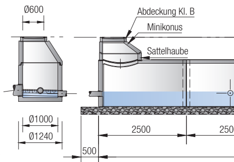
Verteilerschacht
