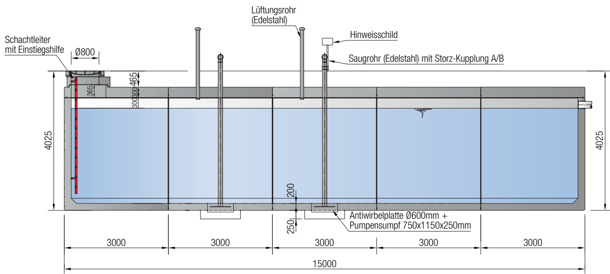
Löschwasserbehälter
