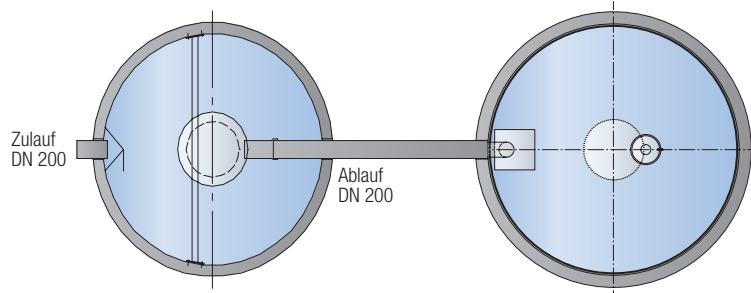
Sickerschacht ViaFil mit Vorfiltervlies und technischem Filter
