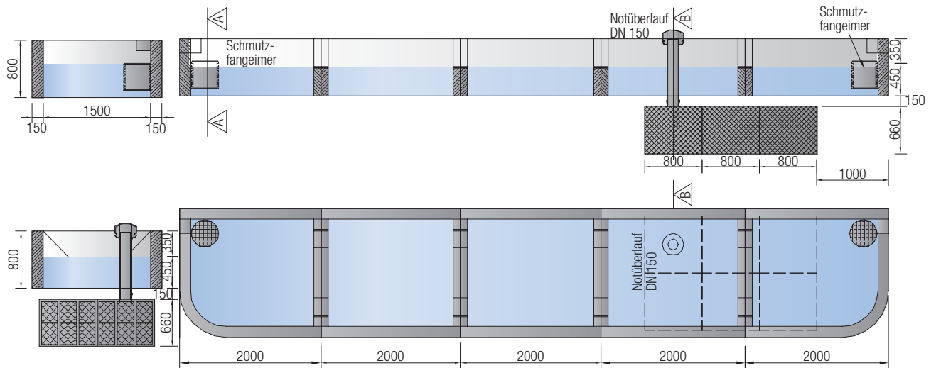
Tiefbeet-Bodenfilter Innodrain
