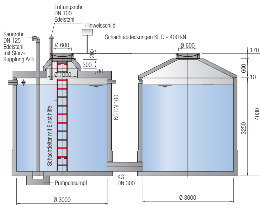
Löschwasserbehälter
