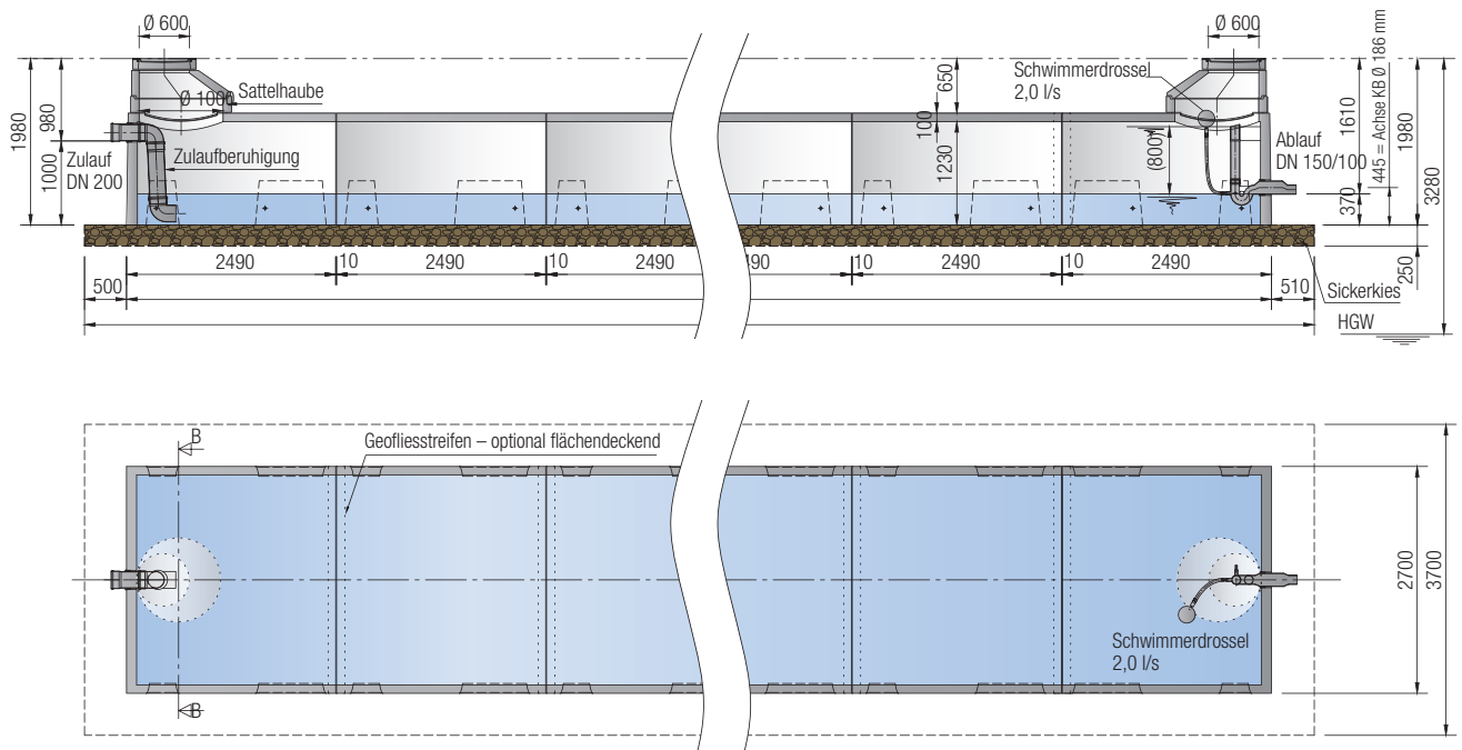
Sickertunnel CaviLine mit Rückhaltung
