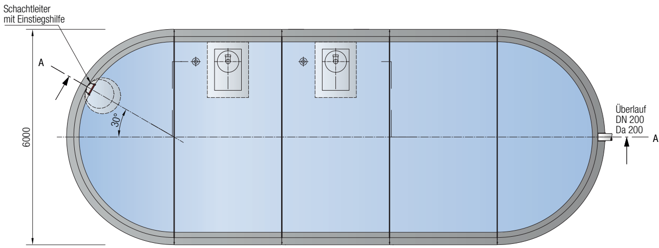
Löschwasserbehälter
