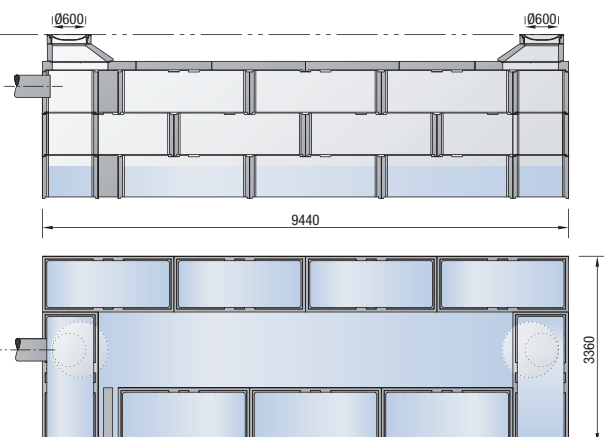
Sickerkammern CaviBox
