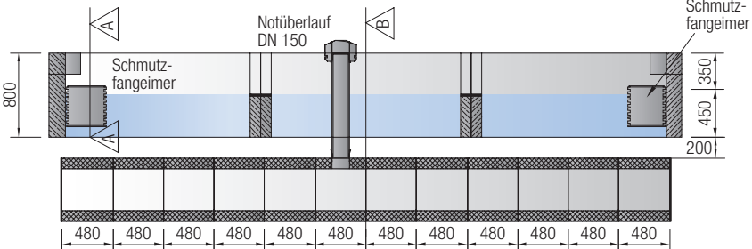
Tiefbeet-Bodenfilter Innodrain
