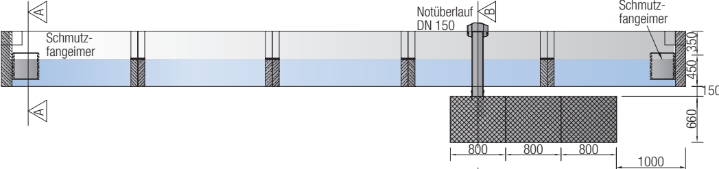
Tiefbeet-Bodenfilter Innodrain
