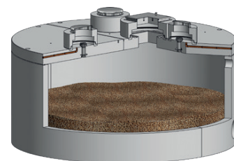
Mall-Pelletspeicher ohne Entnahmesystem von Mall
