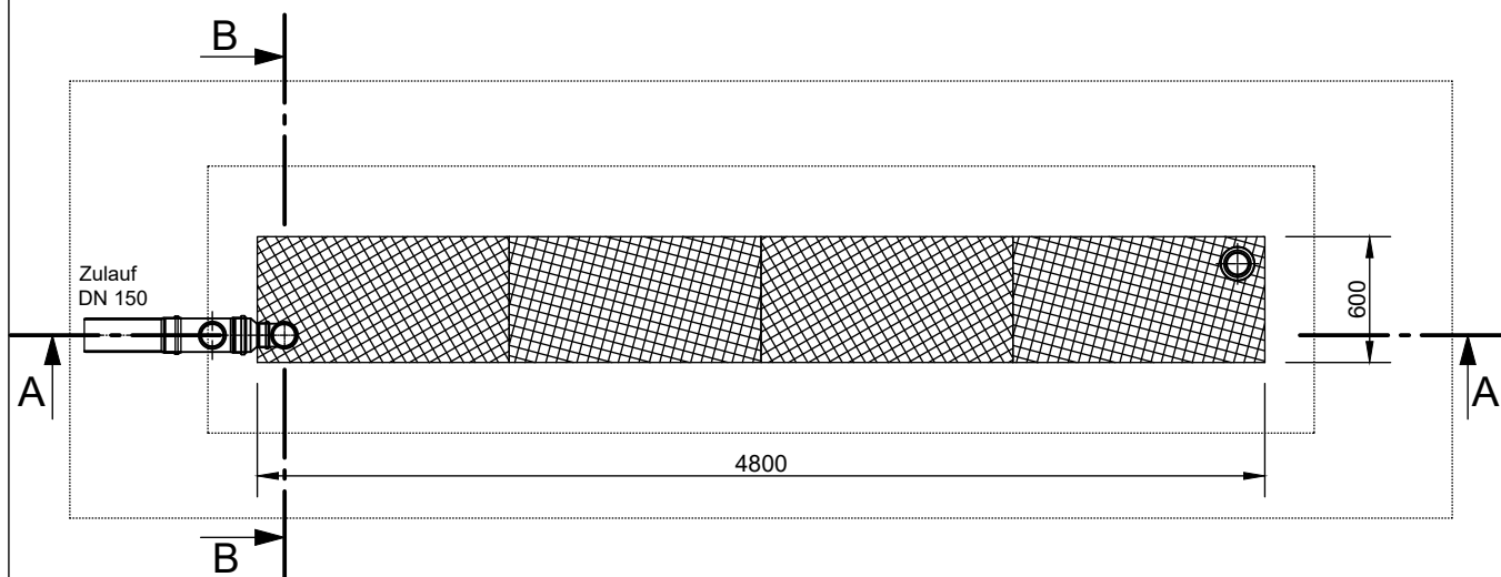
Grundriss
