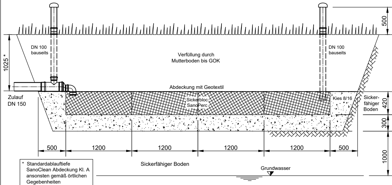
Schnitt A-A
