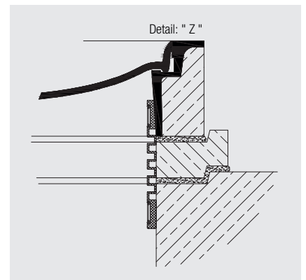
Ringdichtsysteem NeutraProof
