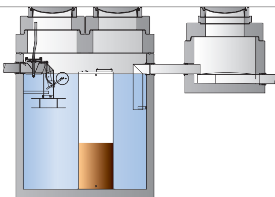
Abscheider Klasse I mit Ölsammelbehälter NeutraPrim
