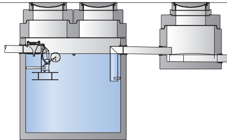
ABKW-Abscheider System A mit Sedimentationseinrichtung NeutraPrim
