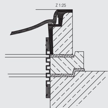
Ringdichtsystem NeutraProof
